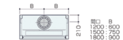
排气管图
