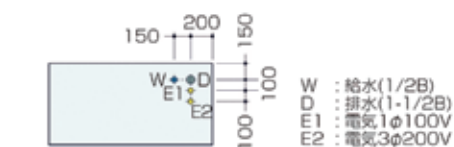
配管图
