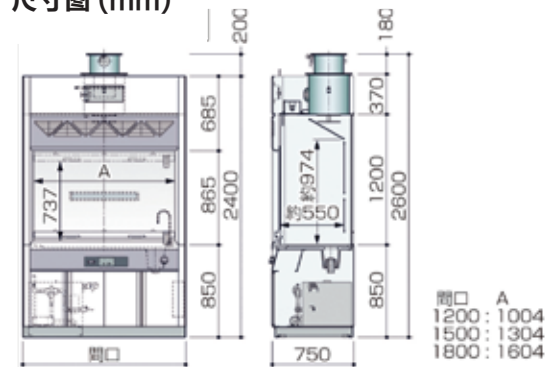
尺寸图 (mm)
